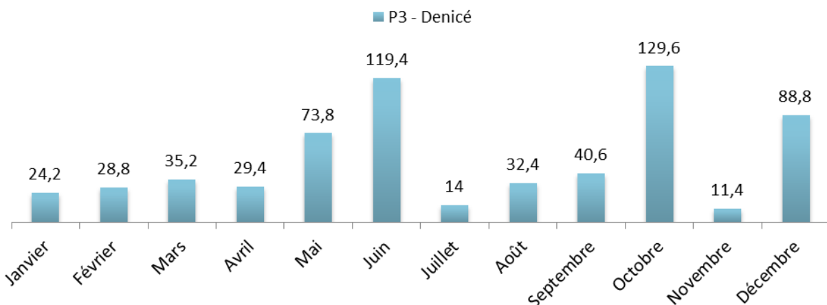
Figure 15 : Evolution mensuelle de la pluviométrie (hauteur précipitée en mm) sur le système de collecte
