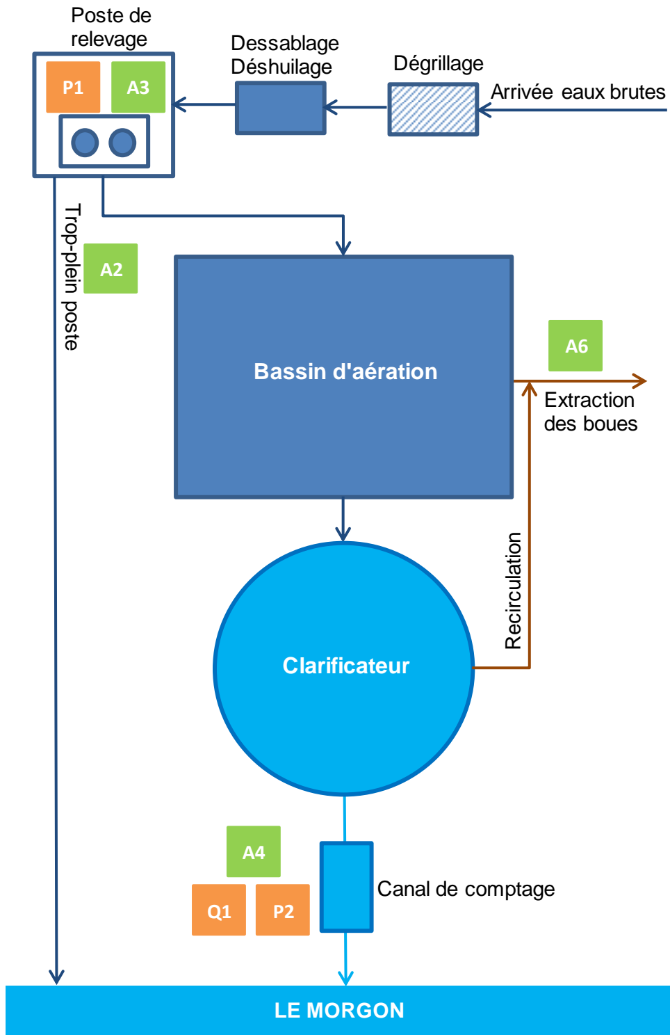
Figure 17 : Synoptique de la station d'épuration actuelle
